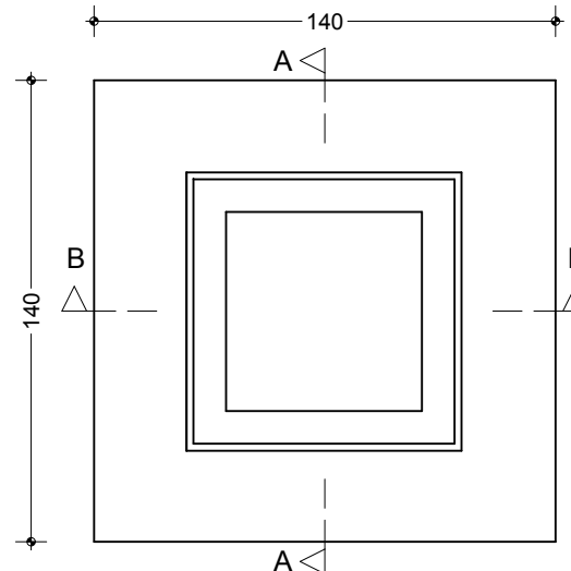
PIANTA COPERCHIO SCALA 1:25
