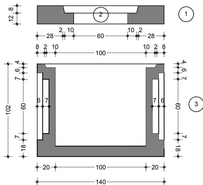
SEZIONE POZZETTO A-A SCALA 1:25
