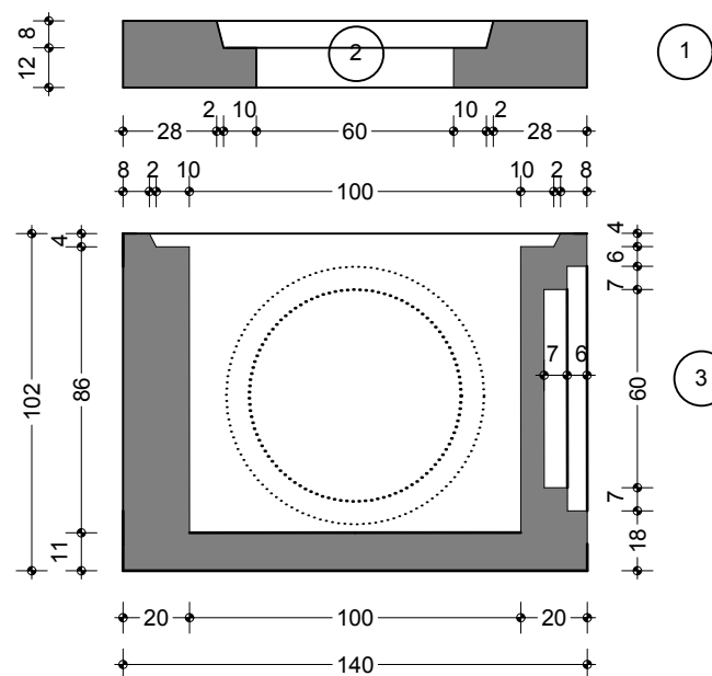
SEZIONE POZZETTO B-B SCALA 1:25
